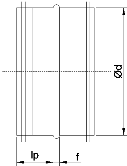
Rysunek 1. Złączka wewnętrzna nypłowa
