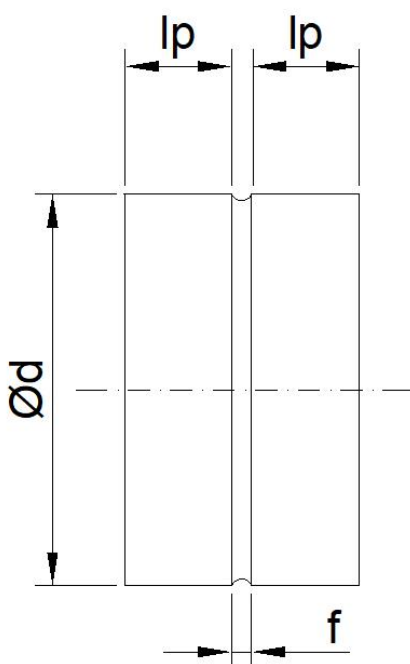
Rysunek 1. Złączka zewnętrzna MF
